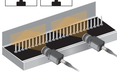
應用於檢測零件印刷
