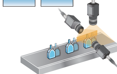
應用於LCD的定位
