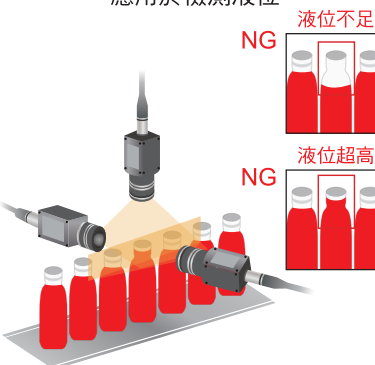
應用於檢測液位
