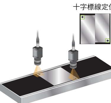
應用於LCD的定位
