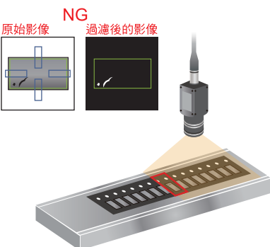
晶片型(SMD)LED的影像檢測
